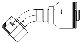
FRA - Female ORS Swivel 45° Elbow
