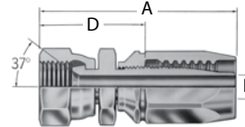
SAE 37° JIC swivel
